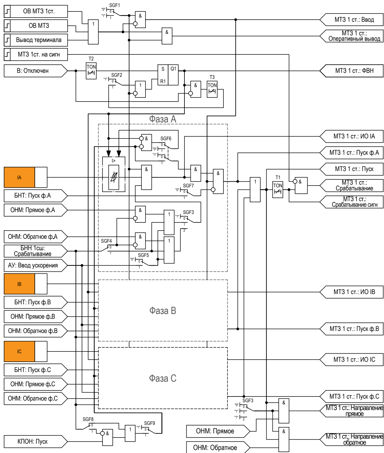
Рисунок 2.13 – Функциональная схема ступени МТЗ
